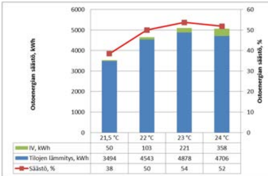
Kuva C6. Realististen ilmalämpöpumppujen ostoenergiansäästö ja sen jakautuminen tilojen ja ilmanvaihdon osuuksiin sekä ostoenergiansäästön osuus tilojen ja ilmanvaihdon lämmöntarpeesta nykyisten määrysten mukaisessa rakennuksessa lämpöpumppujen huonelämpötilan eri asetusarvoilla.
