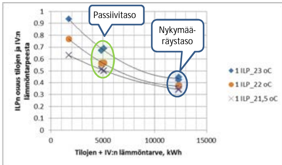
Kuva 16. Ilma-ilmalämpöpumppujen osuus tilojen ja ilmanvaihdon lämmöntarpeesta, kun vain alakerrassa on ilmalämpöpumppu. Osuudet on esitetty ilmalämpöpumpun huonelämpötilan eri asetusarvoilla (21,5 °C, 22 °C ja 23 °C).
