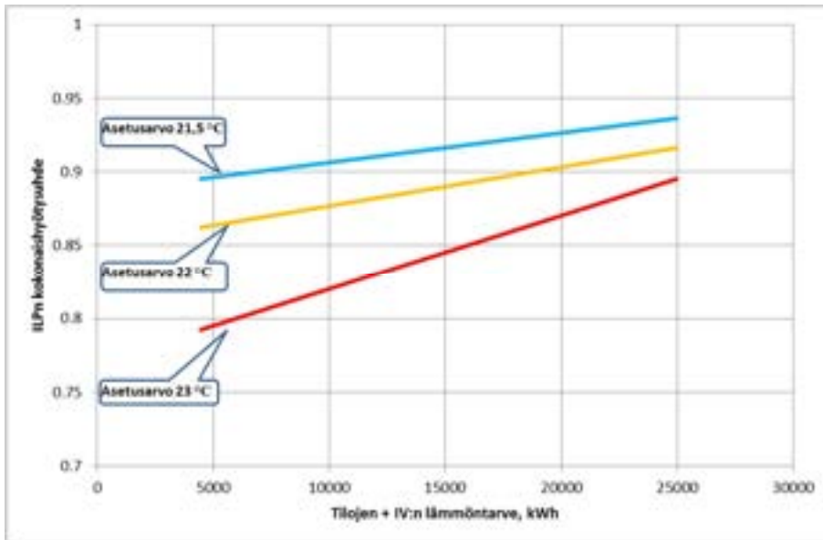
Kuva 29. Ilma-ilmalämpöpumpujen lämmönluovutuksen kokonaishyötysuhde. Kokonaishyötysuhteet on esitetty kolmella eri huonelämpötilan asetusarvolla.
