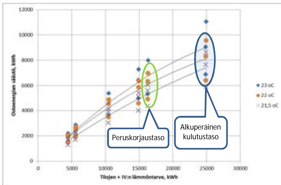
Kuva 27. Ilma-ilmalämpöpumpun ostoenergian säästö. Ostoenergian säästöt on esitetty eri ilmalämpöpumputyypeillä huonelämpötilan asetusarvolla +22 °C.
