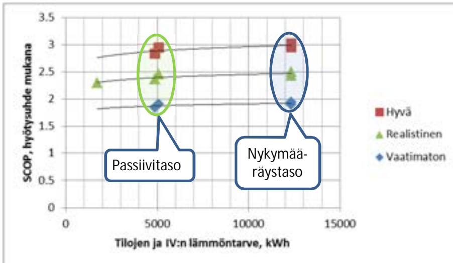
Kuva 23. Ilma-ilmalämpöpumppujen vuotuinen lämpökertoimen, jossa on otettu huomioon ilmalämpöpumpun lämmönluvutuksen kokonaishyötysuhde. Lämpökertoimet on esitetty kolmelle eri lämpöpumpulle (hyvä, realistinen ja vaatimaton) huonelämpötilan asetusarvolla +22 °C.
