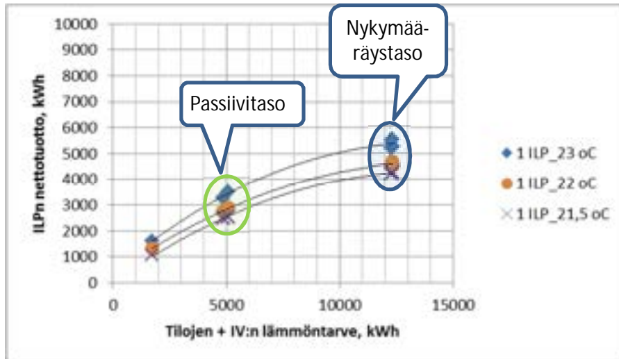
Kuva 15. Ilma-ilmalämpöpumppujen nettotuotto, kun vain alakerrassa on ilmalämpöpumppu. Nettotuotot on esitetty ilmalämpöpumpun huonelämpötilan eri asetusarvoilla (21,5 °C, 22 °C ja 23 °C).
