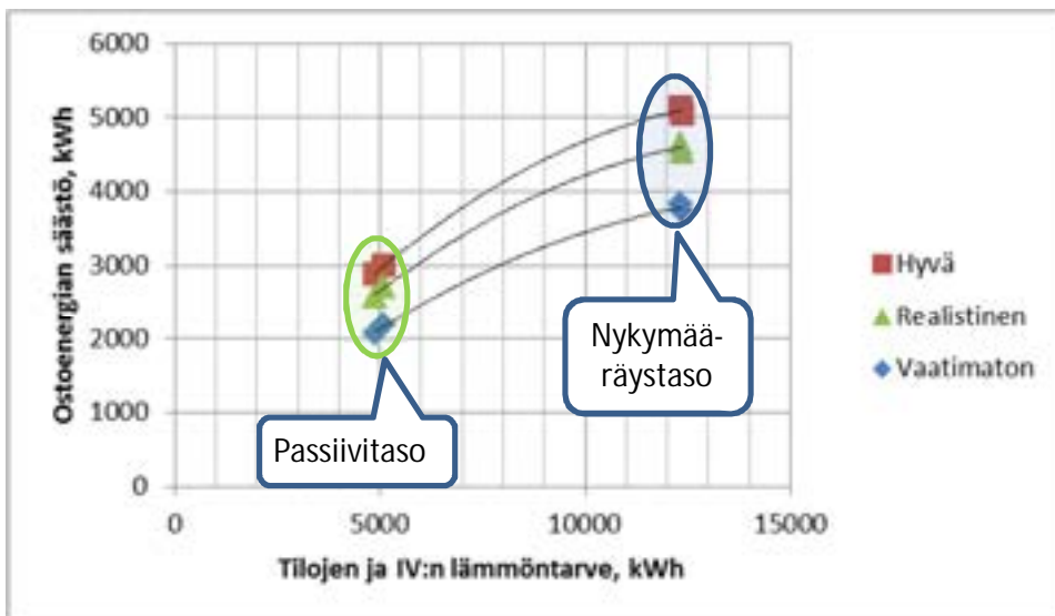
Kuva 20. Ilma-ilmalämpöpumppujen ostoenergian säästö, kun sekä alakerrassa että yläkerrassa on ilma-lämpöpumppu. Ostoenergian säästöt on esitetty eri ilmalämpöpumpputyypeillä huonelämpötilan asetusarvolla +22 °C.
