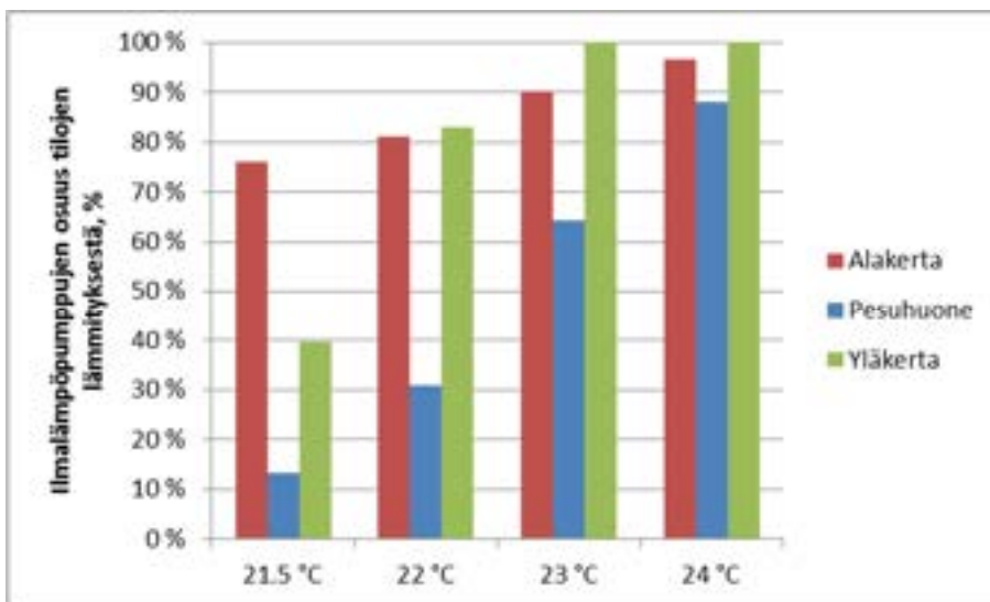
Kuva C7. Realististen ilmalämpöpumppujen osuus tilojen lämmityksestä alakerrassa, erikseen alakerran pesuhuoneessa ja yläkerrassa nykyisten määrysten mukaisessa rakennuksessa lämpöpumppujen huonelämpötilan eri asetusarvoilla.
