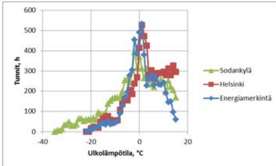
Kuva 11. Simuloinneissa käytetyt säädät Sodankylälle ja Helsingille. Vertailun vuoksi on esitetty myös energiamerkinnässä käytettävä kylmän ilmaston säädäta.
