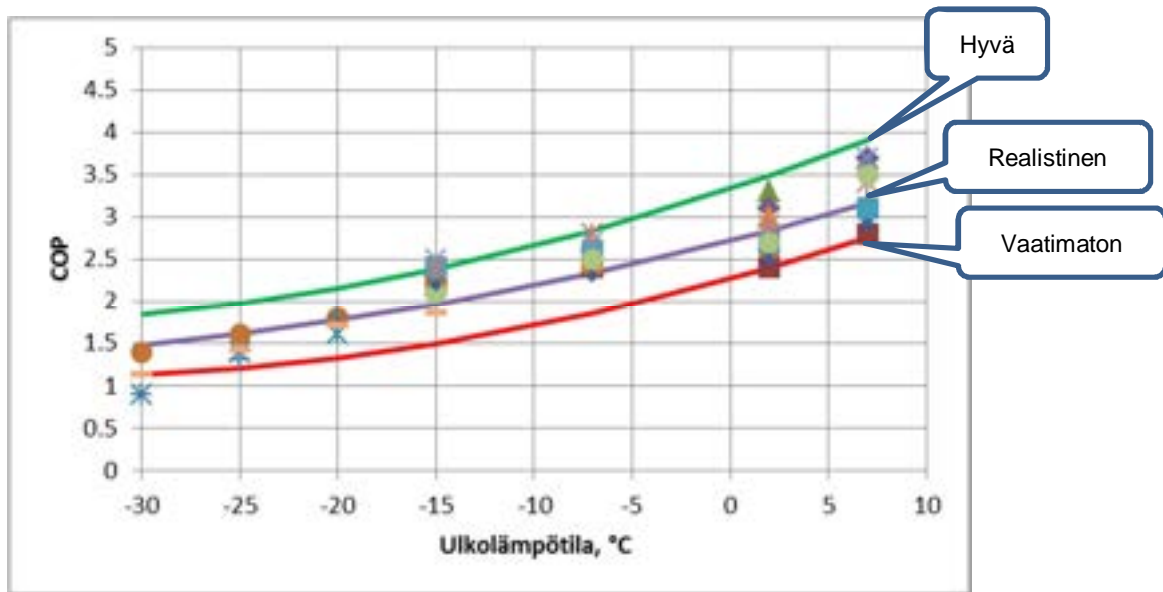
Kuva 6. Simuloinneissa käytetyt ilma-ilmalämpöpumppujen COP-arvot täydellä kuormituksella ulkoilman lämpötilan funktiona. Energimyndighetenin ja Scanoffice Oy:n julkaisemien ilmalämpöpumppujen mittaus tulokset on esitetty kuvassa pisteinä. Sulatuksen sähköenergia sisältyy mitattuihin COP-arvoihin.
