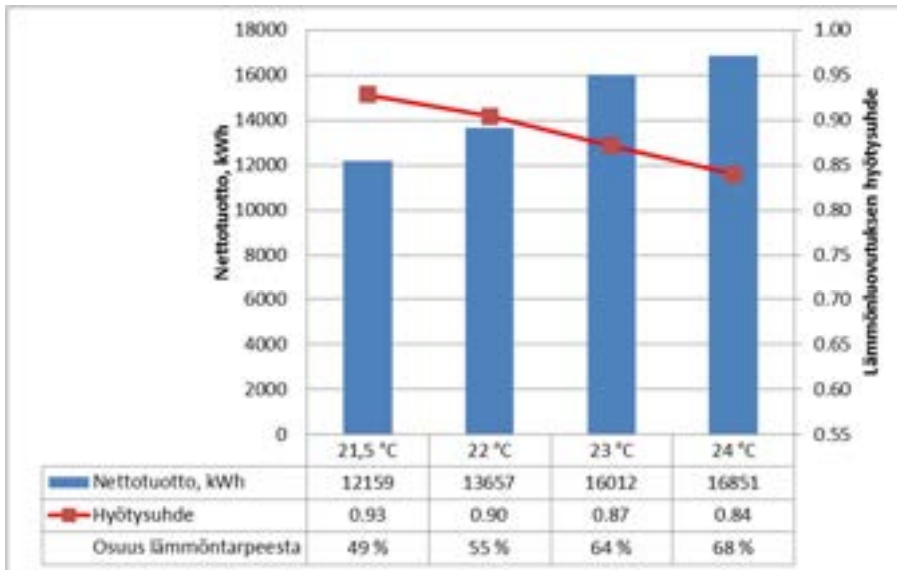
Kuva E4. Realistisen ilmalämpöpumpun nettolämmöntuotto, nettotuoton osuus tilojen ja ilmanvaihdon lämmöntarpeesta ja lämmönluovutuksen kokonaishyötysuhde vanhassa rakennuksessa ilmalämpöpumpun huonelämpötilan eri asetusarvoilla.
