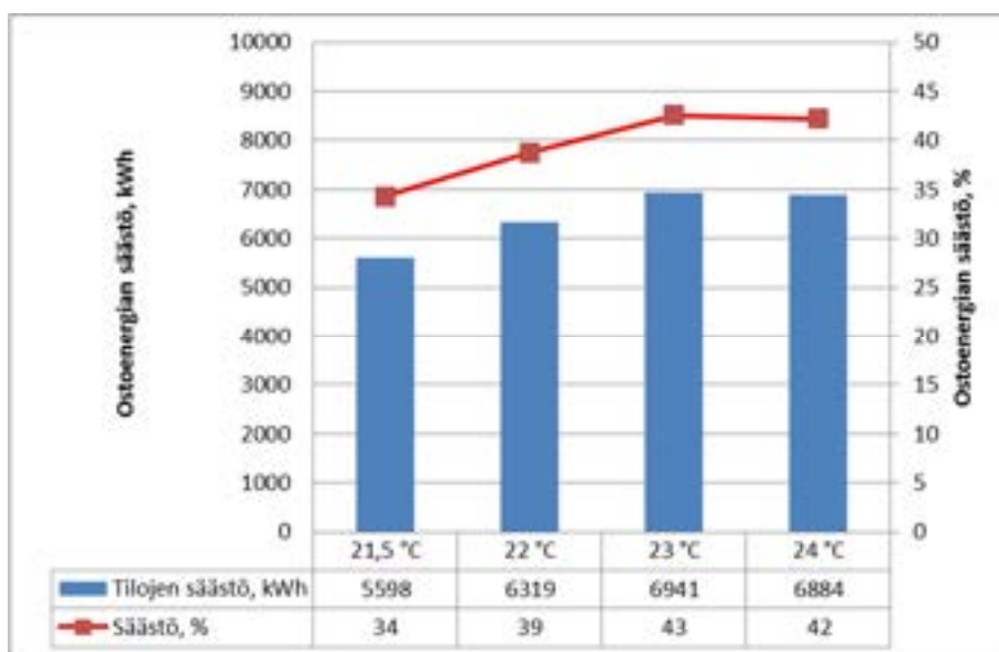
Kuva F5. Realistisen ilmalämpöpumpun ostoenergian säästö sekä ostoenergian säästön osuus tilojen ja ilmanvaihdon lämmöntarpeesta vanhassa rakennuksessa ilmalämpöpumpun huonelämpötilan eri asetusarvoilla.
