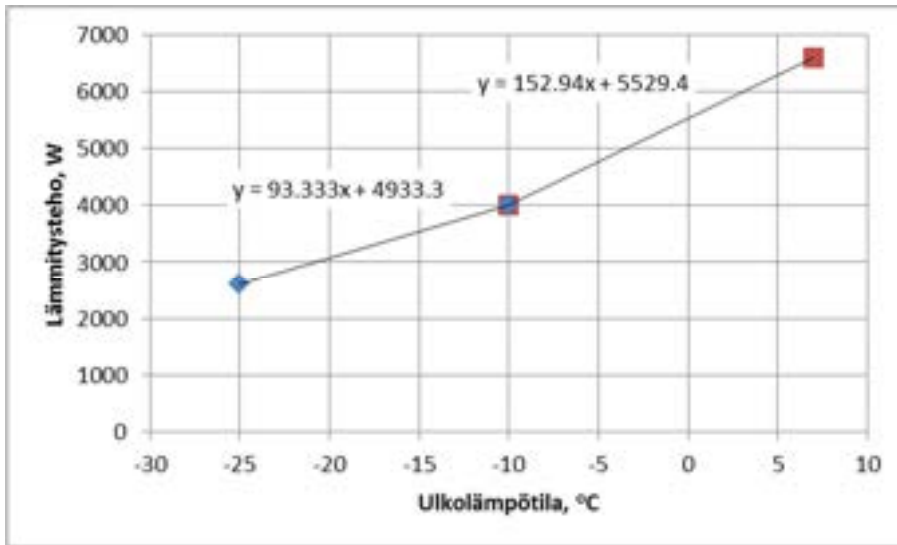
Kuva G1. Ilma-ilmalämpöpumpun lämmitysteho (taulukko G1) ulkoilman lämpötilan funktiona sekä interpoloinneissa ja ekstrapoloinnissa käytetyt lineaariset sovitteet.
