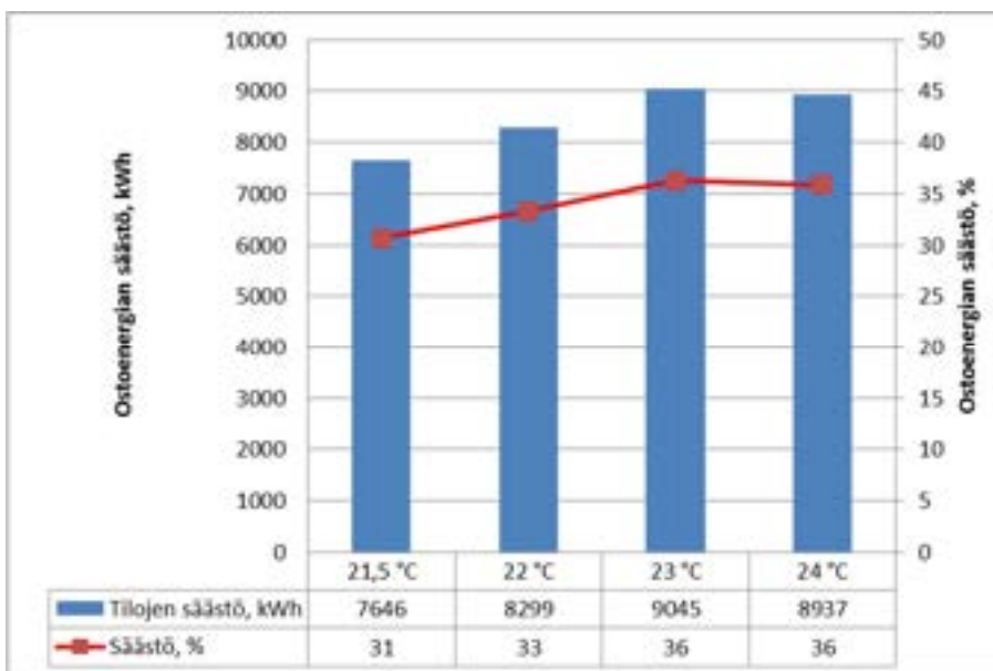
Kuva E5. Realistisen ilmalämpöpumpun ostoenegiansäästö sekä ostoenegiansäästön osuus tilojen ja ilmanvaihdon lämmöntarpeesta vanhassa rakennuksessa ilmalämpöpumpun huonelämpötilan eri asetusarvoilla.
