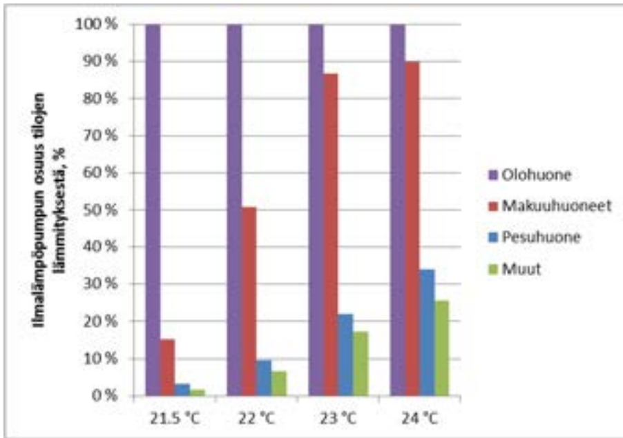
Kuva F6. Realistisen ilmalämpöpumpun osuus tilojen lämmityksestä vanhassa rakennuksessa lämpöpumpun huonelämpötilan eri asetuservoilla.
